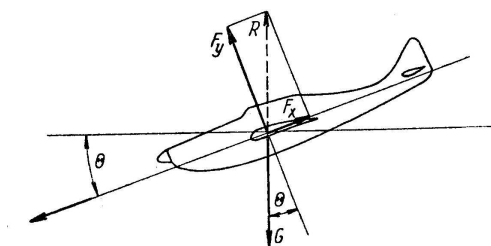
Obr. 28 Letadlo při rovnoměrném klouzavém letu
