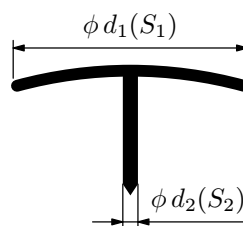
Obr. 7 Řez připínáčkem
