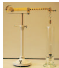
Obr. 45 Mohrovy vážky
