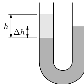
Obr. 23 U-trubice
