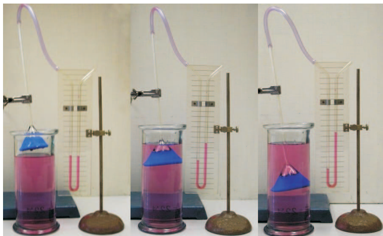
Obr. 55 Výroba manometru
