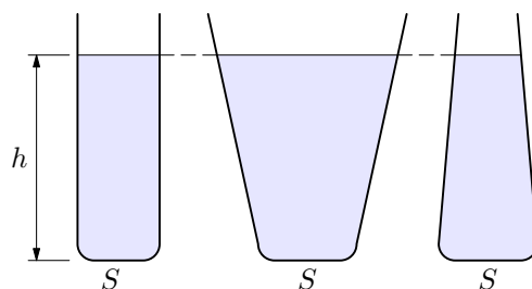
Obr. 13 Hydrostatické paradoxon
