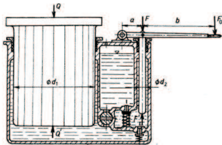
Obr. 10 Hydraulický zvedák
