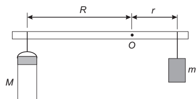
Obr. 42 Pravitko
