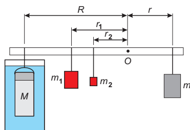
Obr. 44 Obnovení rovnováhy
