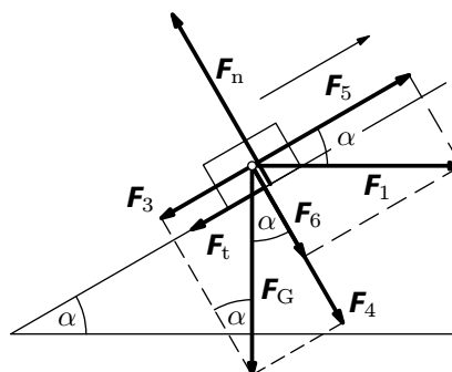
Obr. 20 Rozklad sil
