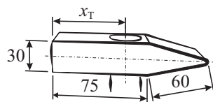
Obr. 48 Kladivo
