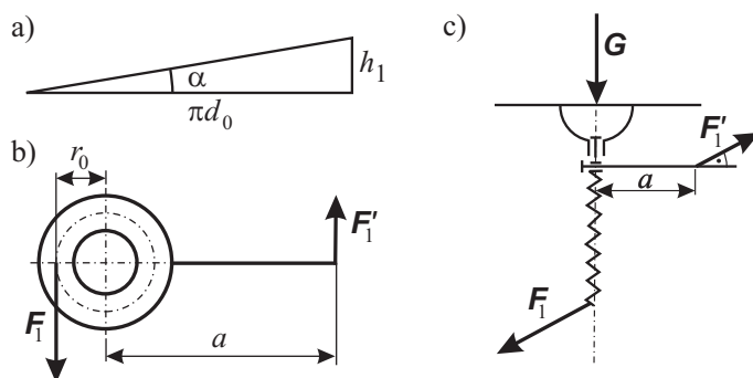
Obr. 22 Šroubový zdvihák 2
