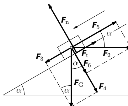
Obr. 52 Rozklad sil
