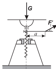
Obr. 21 Šroubový zdvihák 1
