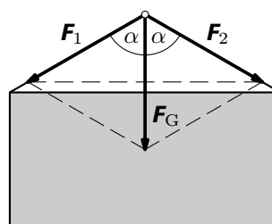
Obr. 54 Závěšení břemene
