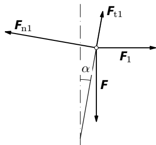
Obr. 53 Rozklad sil
