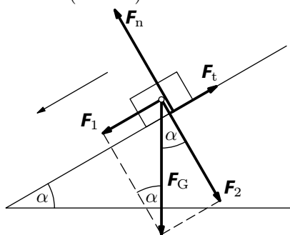
Obr. 15 Nakloněná rovina – pohyb samovolně směrem dolů
