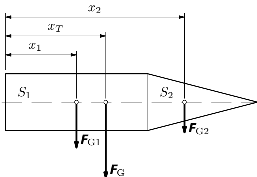
Obr. 57 Kladívko
