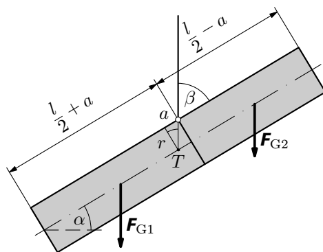
Obr. 56 Zavěšená roura
