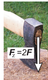
Obr. 25 Štípání sekyrkou
