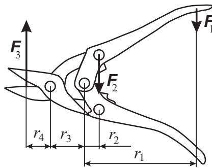
Obr. 8 Nůžky na plech – síly
