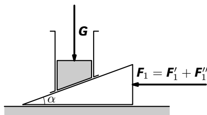
Obr. 23 Zarážení klínu
