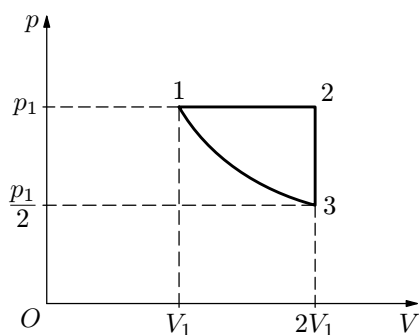
Obr. 8 Děj [3 \rightarrow 1] je izotermický.
