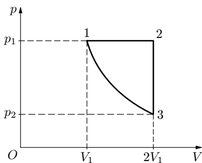
Obr. 9 Děj [3 \rightarrow 1] je adiabatický.
