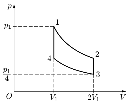
Obr. 10 Děje [1 \rightarrow 2] a [3 \rightarrow 4] jsou izotermické.
